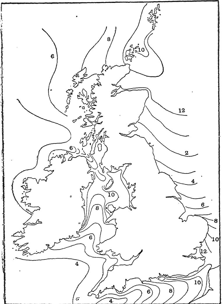
चित्र ८५—प्रगामी तरंग के सिद्धान्त के अनुसार ब्रिटिश समुद्र में अनुरूप ज्वारभाटा की रेखाएँ ।
